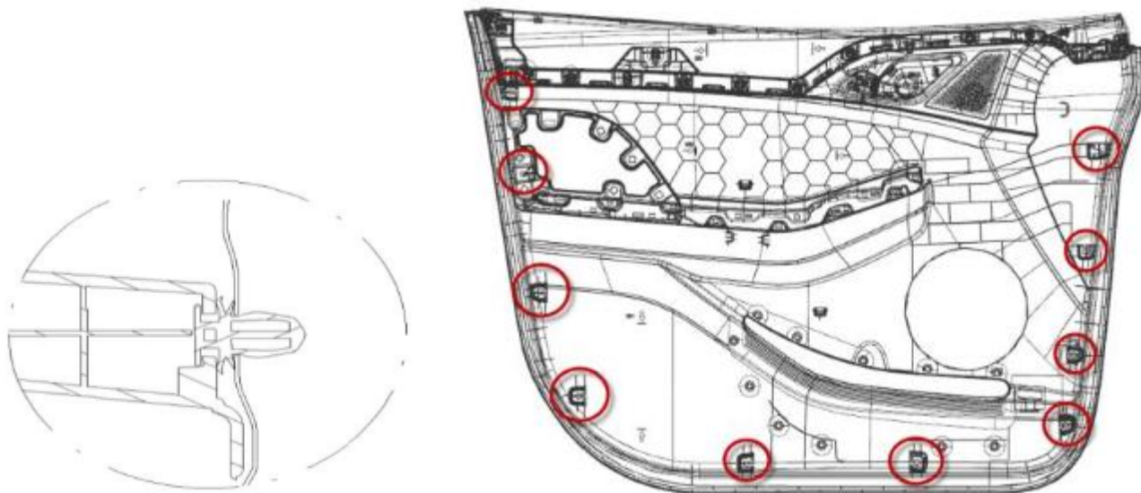
Рисунок 3 Схематическое изображение положения пластиковой пряжки
